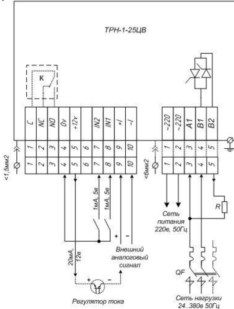
Рисунок 3. Схема подключения.
